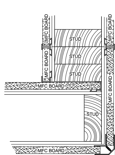
STUD PARTITION CORNER SECTION G.A.
